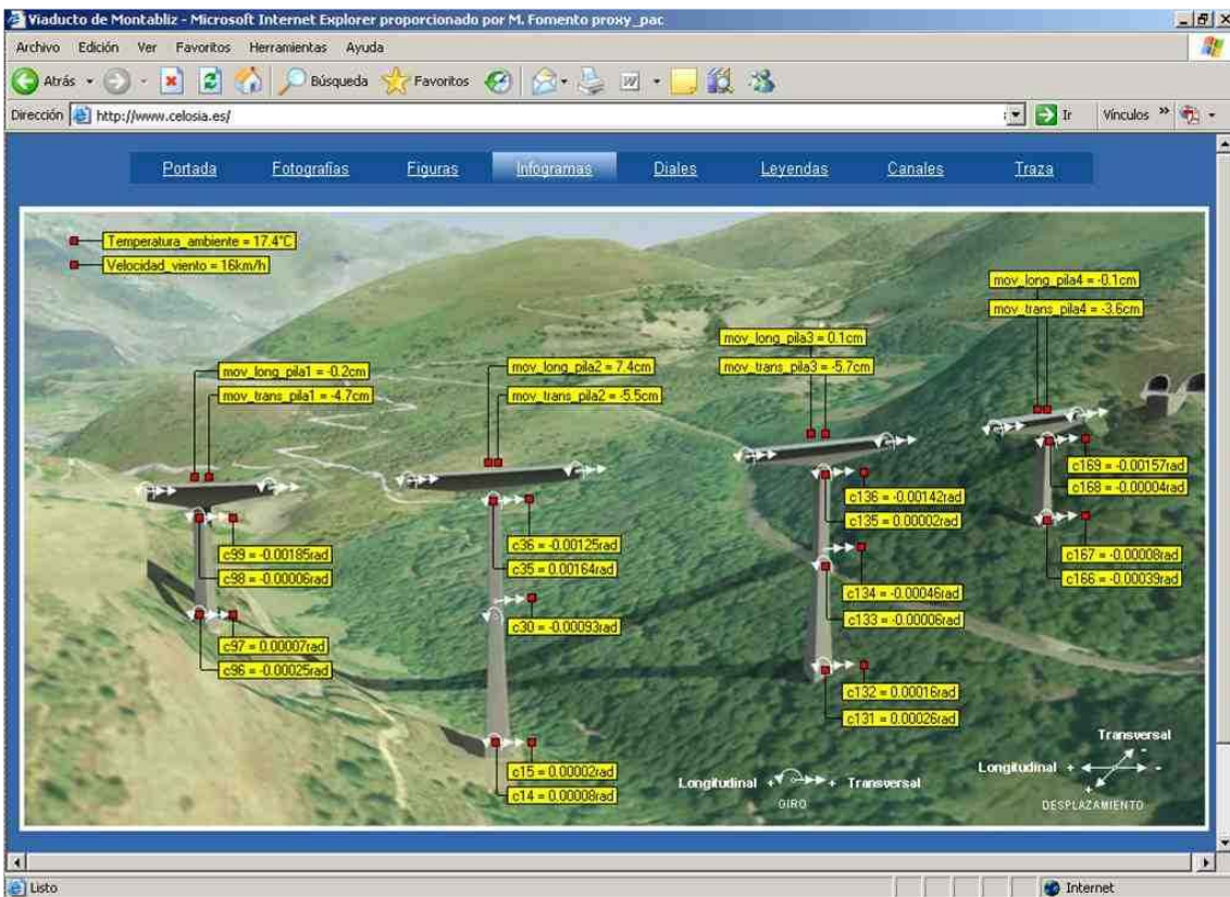
Figura 6- Infograma para control de giros y movimientos en pilas (Viaducto de Montabliz)
