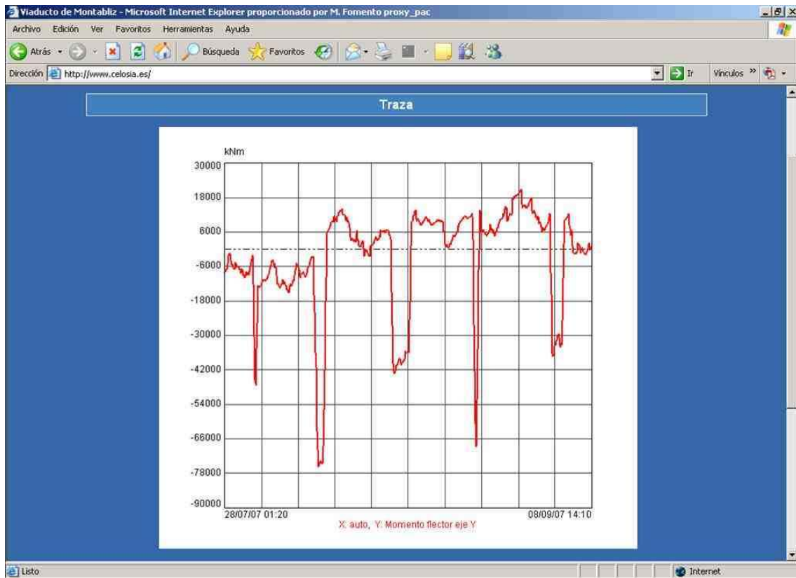
Figura 7 - Variación del momento flector en base de pila producida por el hormigonado de cinco semi-dovelas de tablero del brazo Norte y sus cinco semi-dovelas equivalentes del brazo Sur (Viaducto de Montabliz)
