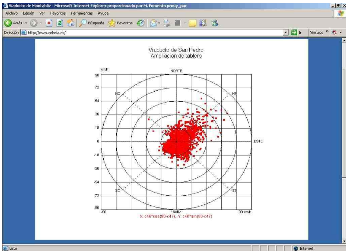
Figura 8 - Diagrama polar de viento para limitación de operaciones constructivas (San Pedro)
