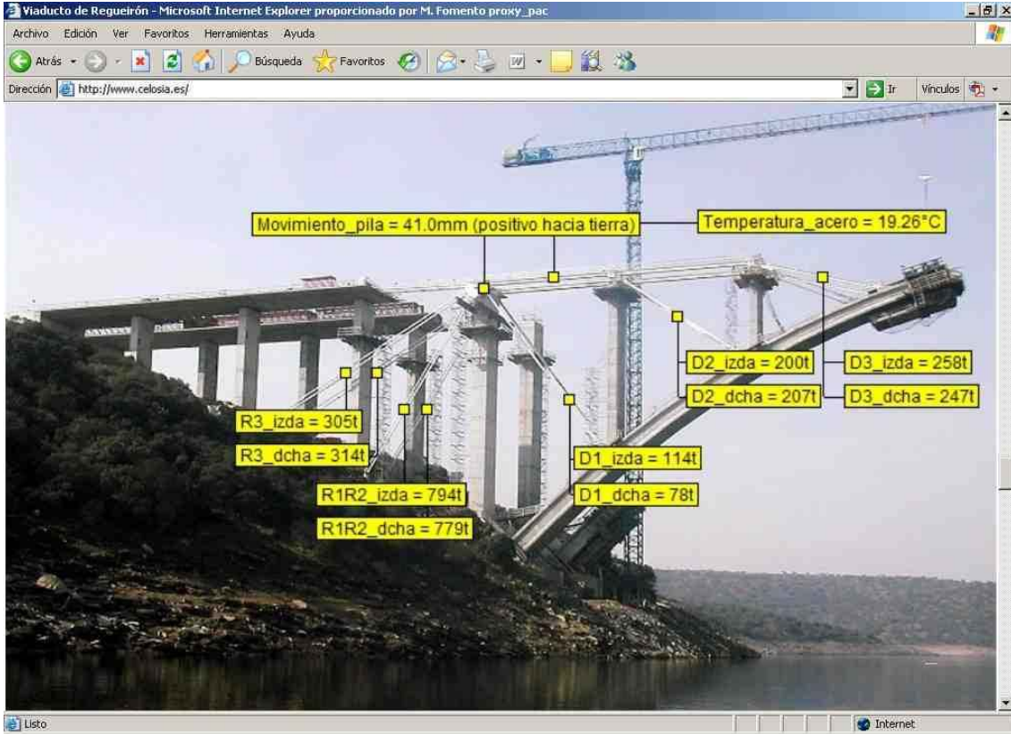
Figura 5 - Infograma para control de fuerzas en tirantes y movimientos en pilas (Viaducto de Almonte)
