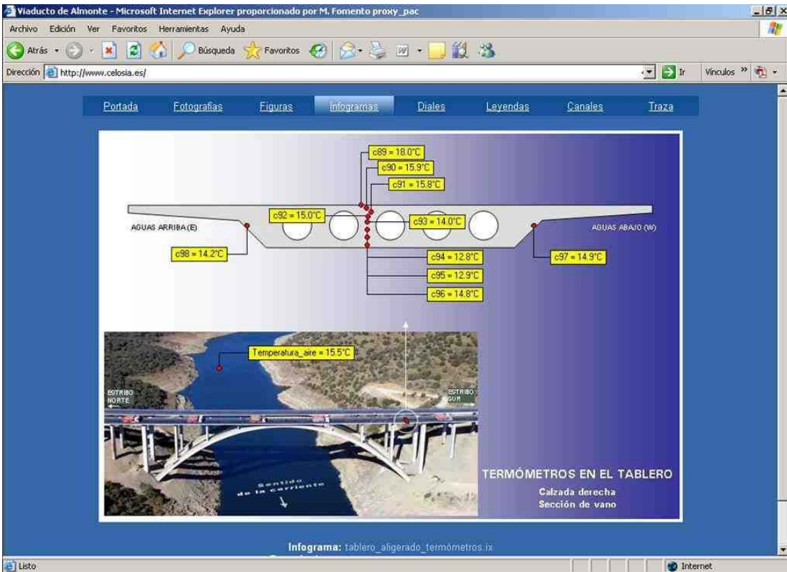
Figura 12 - Infograma para estudio térmico del tablero (Viaducto de Almonte)
